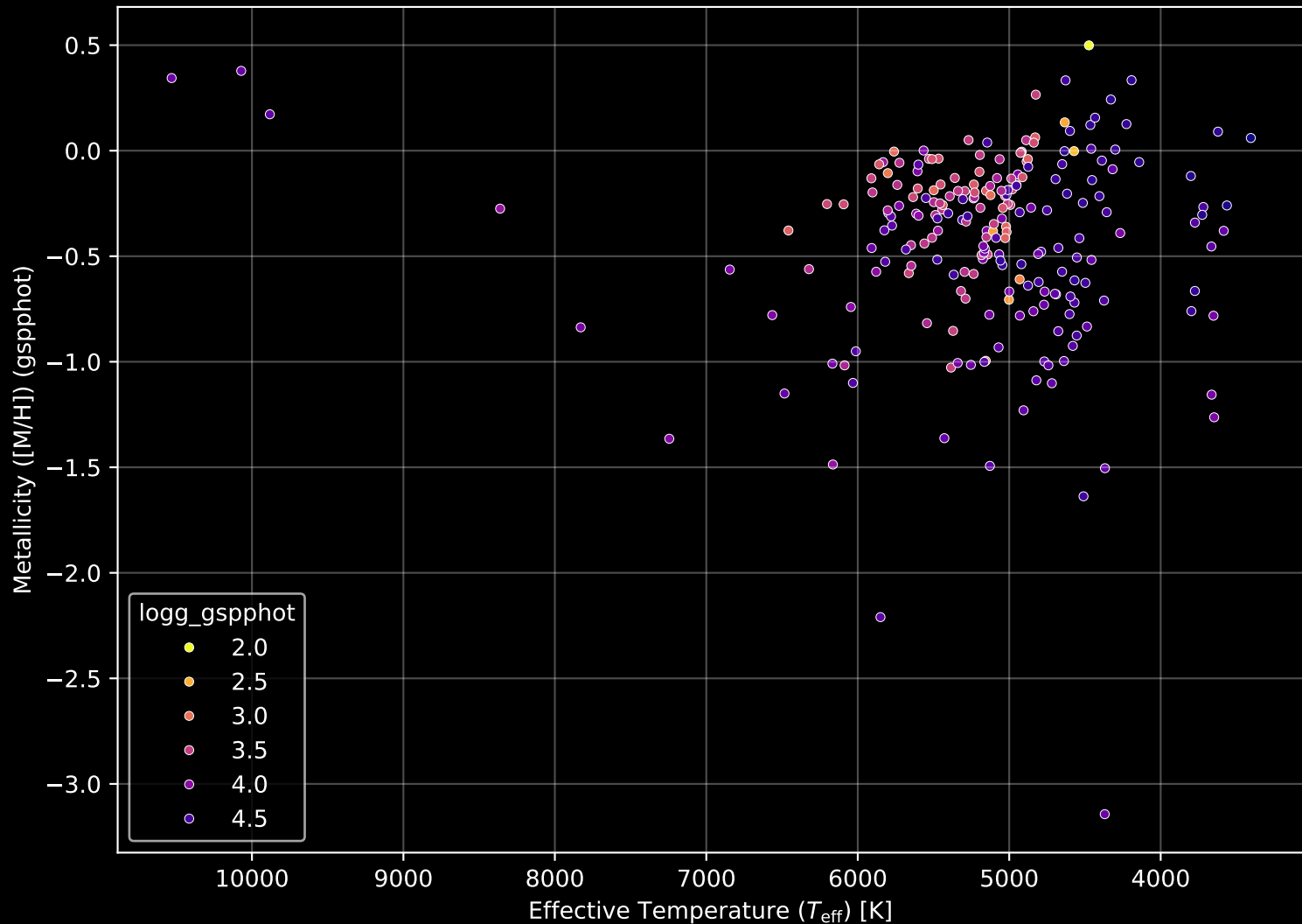
APOGEE DR17 Field: [291-25-C] Stellar Population Parameters (n= 224)
